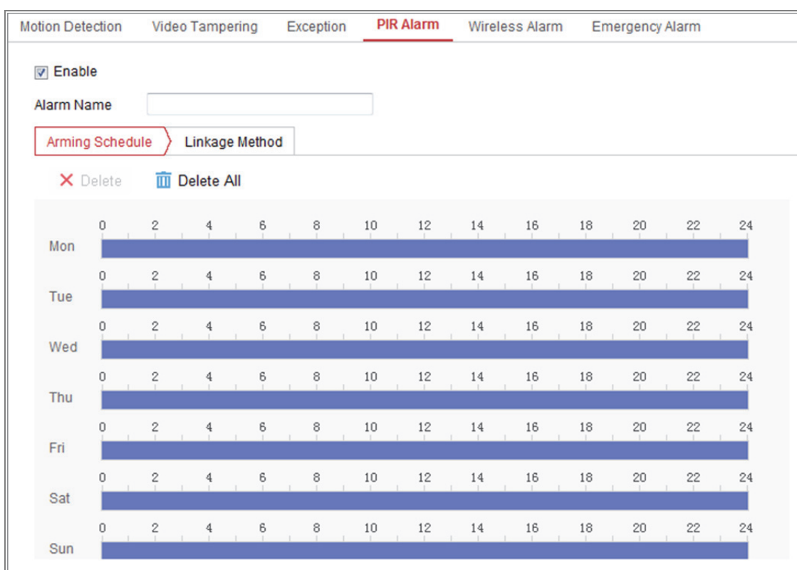
Obrázek 10-12 Nastavení alarmu PIR
