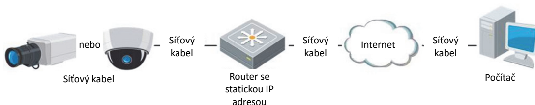
Obrázek 2-10 Přístup ke kameře prostřednictvím směrovače se statickou IP adresou
