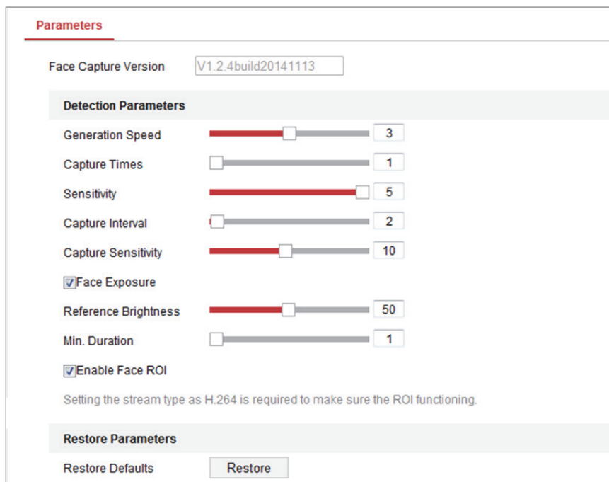
Obrázek 10-30 Pokročilá konfigurace snímání obličeje
