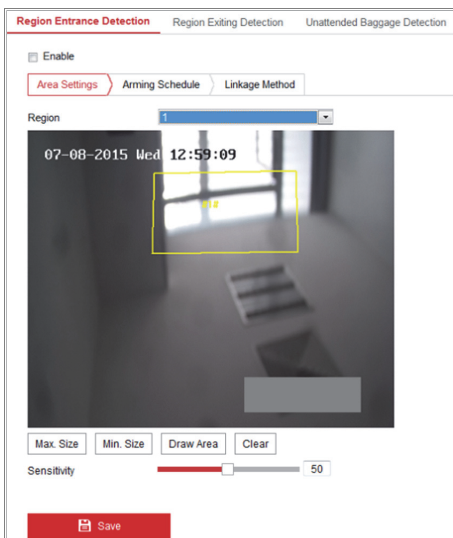
Obrázek 10-21 Detekce vstupování do oblasti
