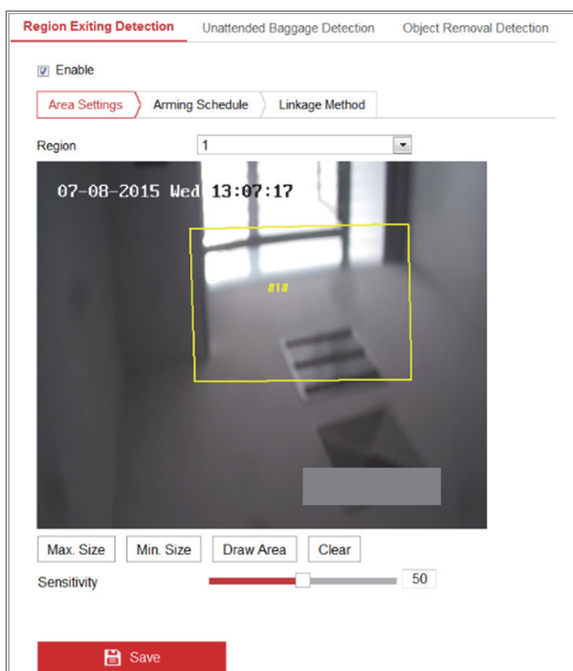
Obrázek 10-22 Detekce vystupování z oblasti
