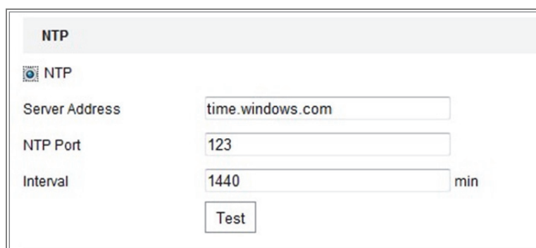
Obrázek 6-4 Synchronizace času podle serveru NTP
