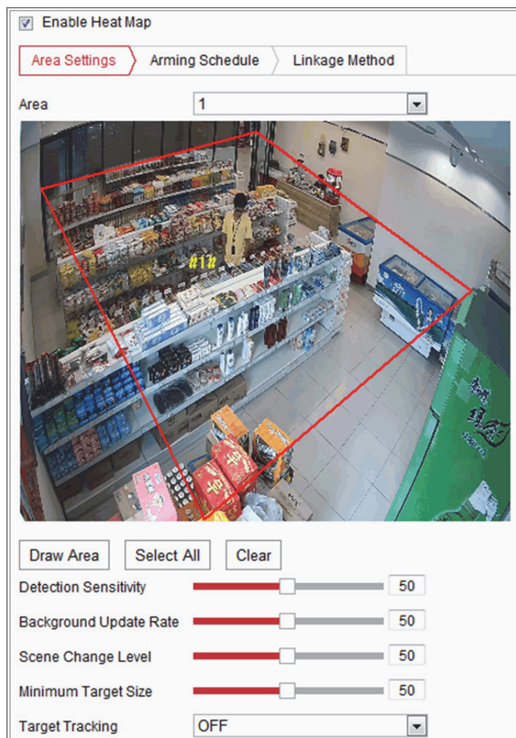
Obrázek 10-34 Konfigurace tepelné mapy
