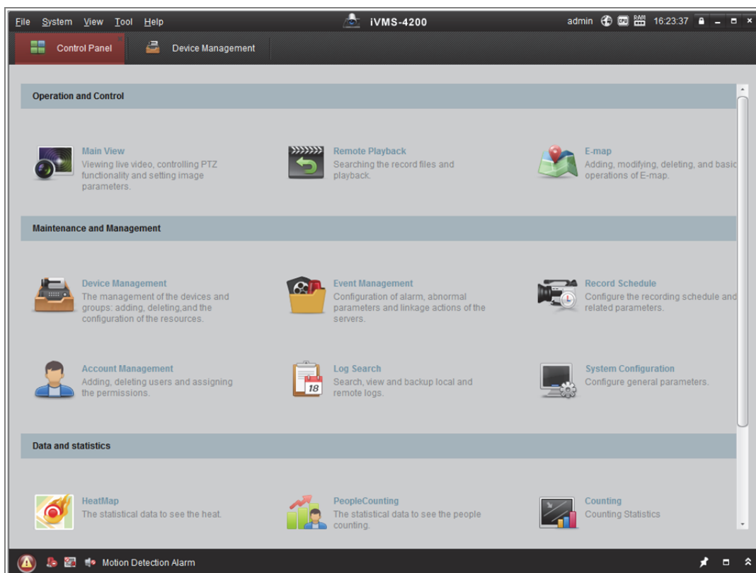
Obrázek 3-2 Ovládací panel iVMS-4200
