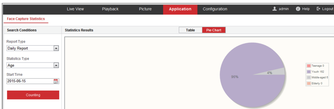
Obrázek 14-1 Okno použití
